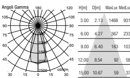
PEGASO 3 40° - 70W - 3000K
