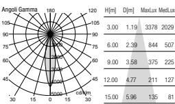
PEGASO 3 20° - 70W - 3000K
