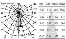
PEGASO 4 20° - 90W - 3000K
