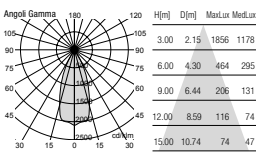
PEGASO 4 40° - 90W - 3000K
